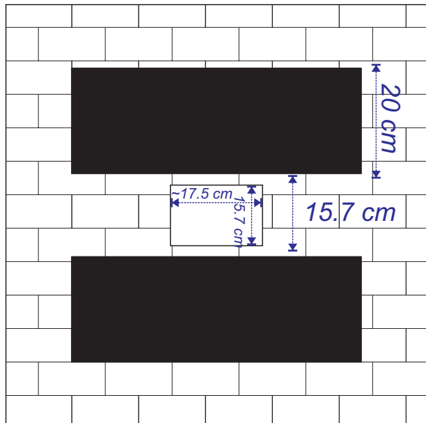
Front view PE wall
