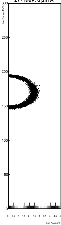
277 MeV, 8 \mu\text{m} Al
