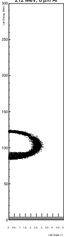
212 MeV, 8 \mu\text{m} Al
