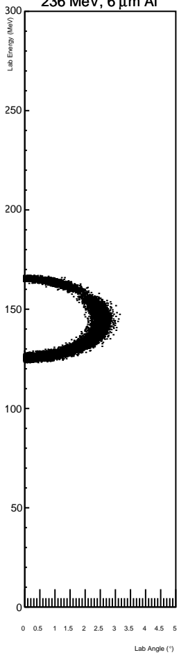
236 MeV, 6 \mu\text{m} Al
