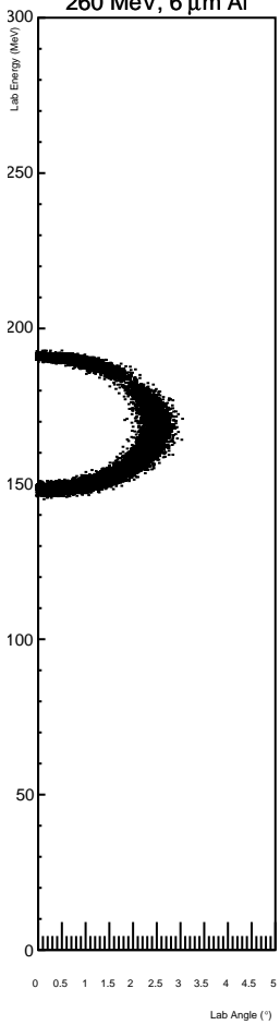
260 MeV, 6 \mu\text{m} Al
