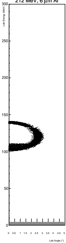
212 MeV, 6 \mu\text{m} Al
