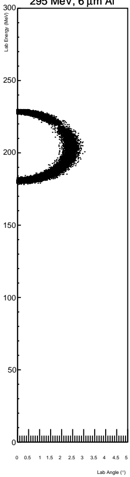
295 MeV, 6 \mu\text{m} Al
