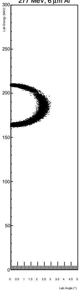
277 MeV, 6 \mu\text{m} Al
