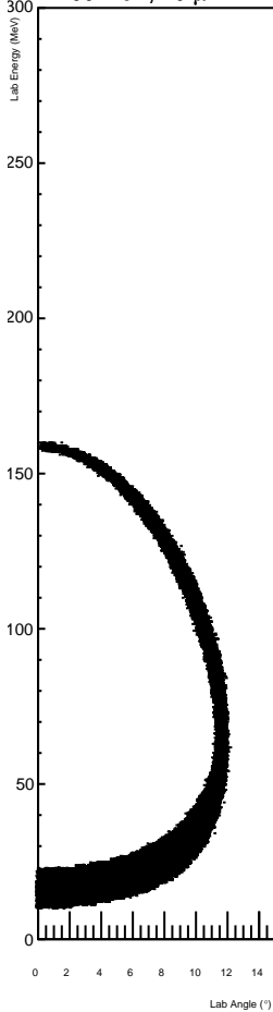
260 MeV, 10 \mu\text{m} Al
