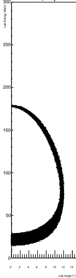
277 MeV, 10 \mu\text{m} Al
