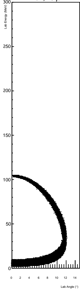
212 MeV, 10 \mu\text{m} Al
