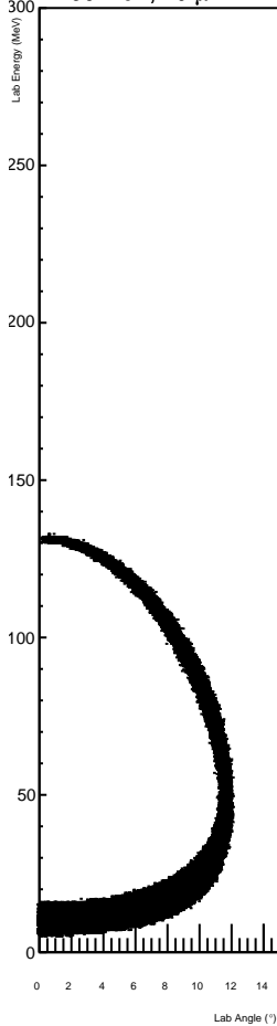
236 MeV, 10 \mu\text{m} Al
