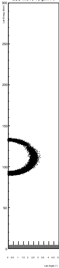
236 MeV, 10 \mu\text{m} Al
