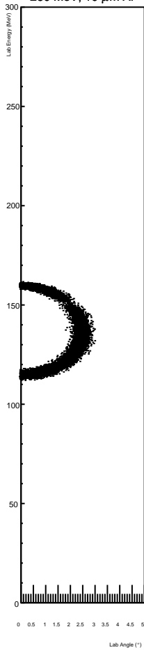
260 MeV, 10 \mu\text{m} Al
