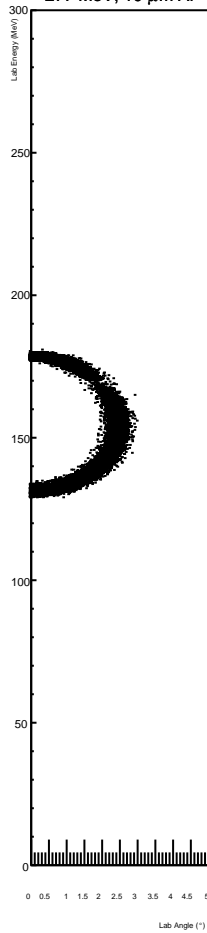
277 MeV, 10 \mu\text{m} Al
