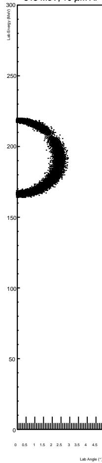
313 MeV, 10 \mu\text{m} Al
