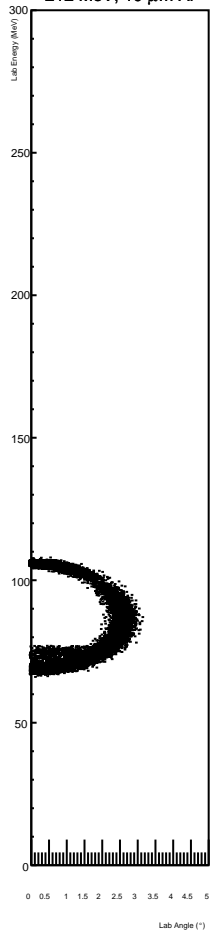
212 MeV, 10 \mu\text{m} Al
