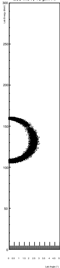
295 MeV, 15 \mu\text{m} Al
