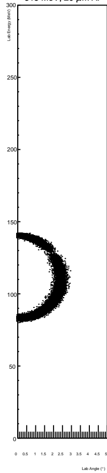
313 MeV, 20 \mu\text{m} Al
