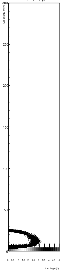
212 MeV, 20 \mu\text{m} Al
