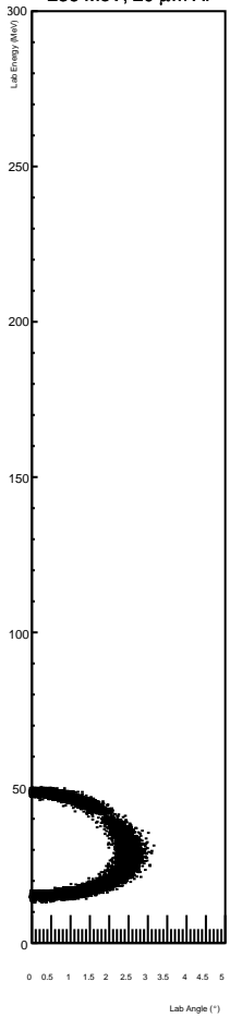
236 MeV, 20 \mu\text{m} Al
