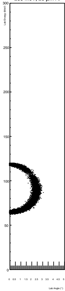
295 MeV, 20 \mu\text{m} Al
