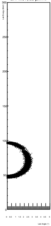
277 MeV, 20 \mu\text{m} Al
