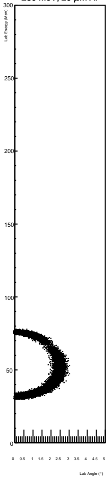
260 MeV, 20 \mu\text{m} Al
