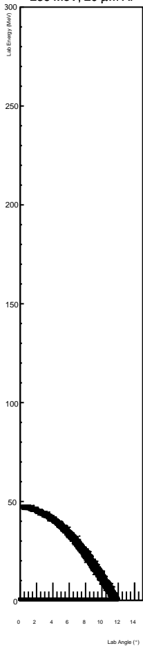
236 MeV, 20 \mu\text{m} Al
