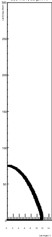
260 MeV, 20 \mu\text{m} Al
