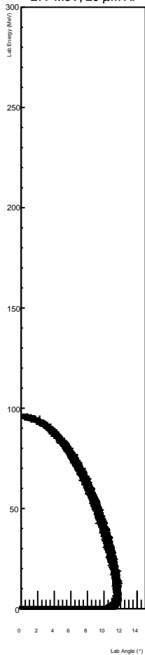
277 MeV, 20 \mu\text{m} Al
