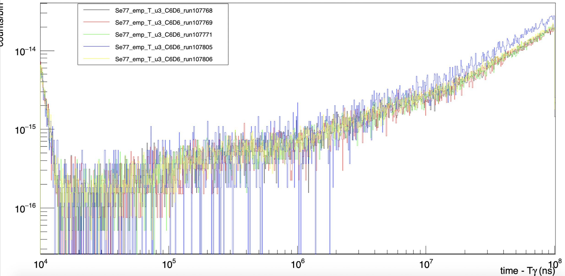
Se77_emp_T_u3_C6D6_run107768
