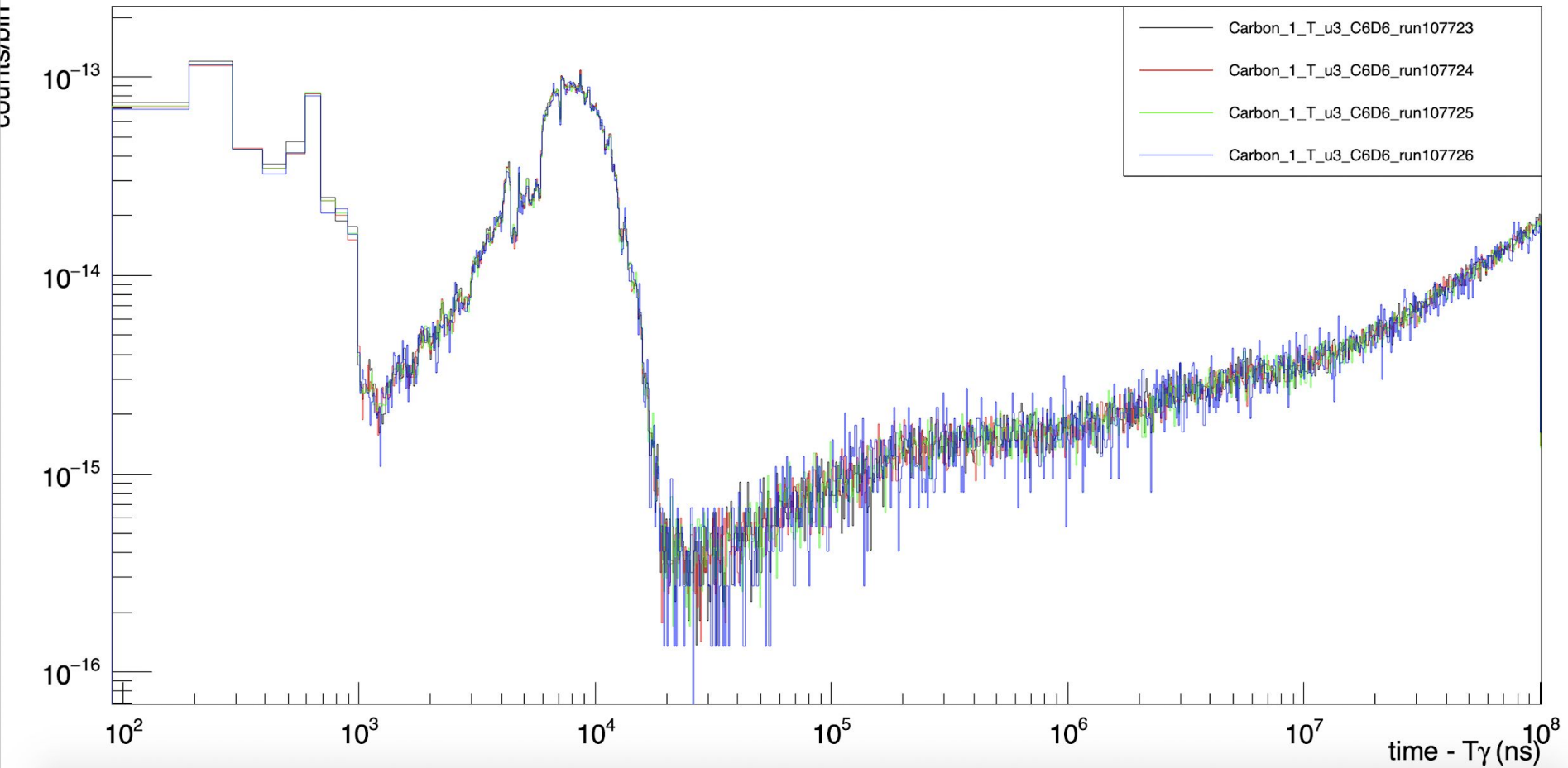
Carbon_1_T_u3_C6D6_run107723
