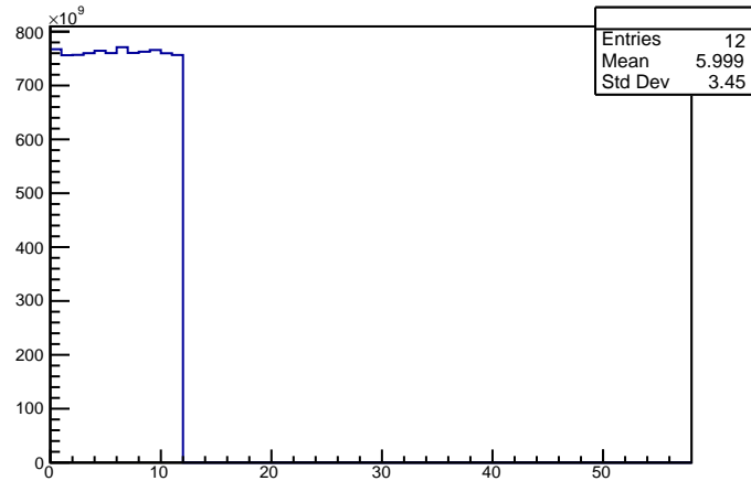
SILI
