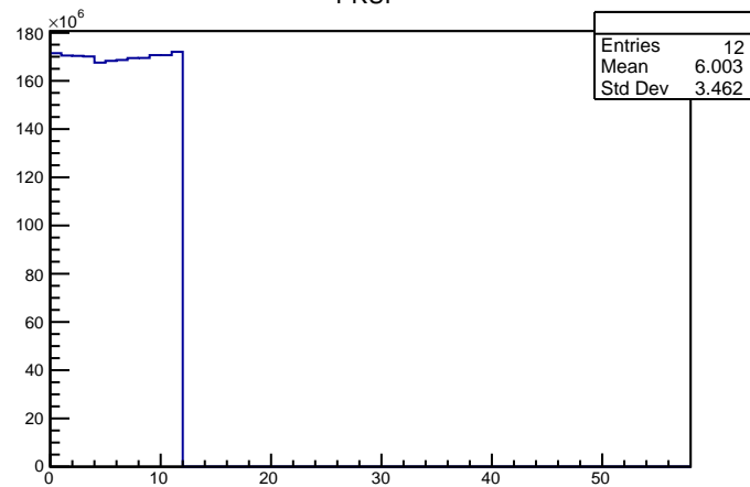
PKUP
